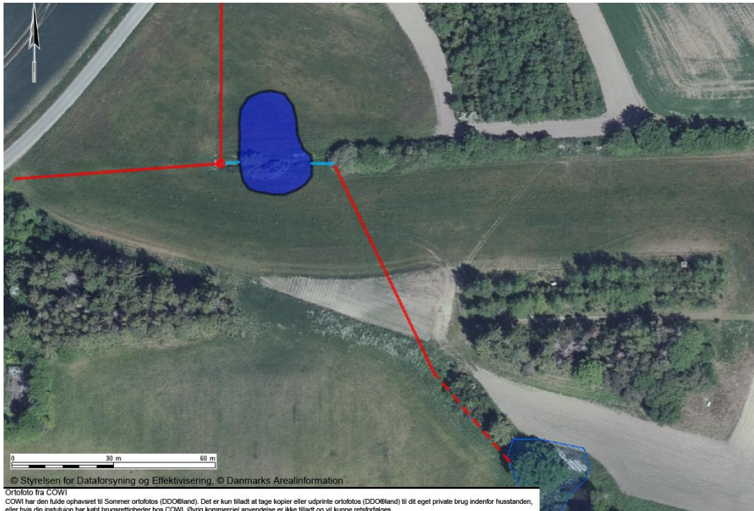
Figur 3. Dræn og grøfter efter etablering af vandhul (rød streg angiver drænløsnings, rød stiptet streg angiver åbne grøfter, rød cirkel angiver eksisterende overløbsbrønd, lyseblå streg angiver ny drænløsnings. Eksisterende sø ses mod sydøst. Vand afledes mod nord.
