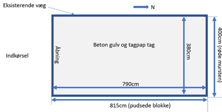
Tegning 1 - Længde og bredde på den ansøgte carport.
