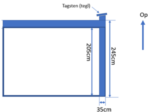
Tegning 2 - Carporten set foran hvor højdemål er angivet.
